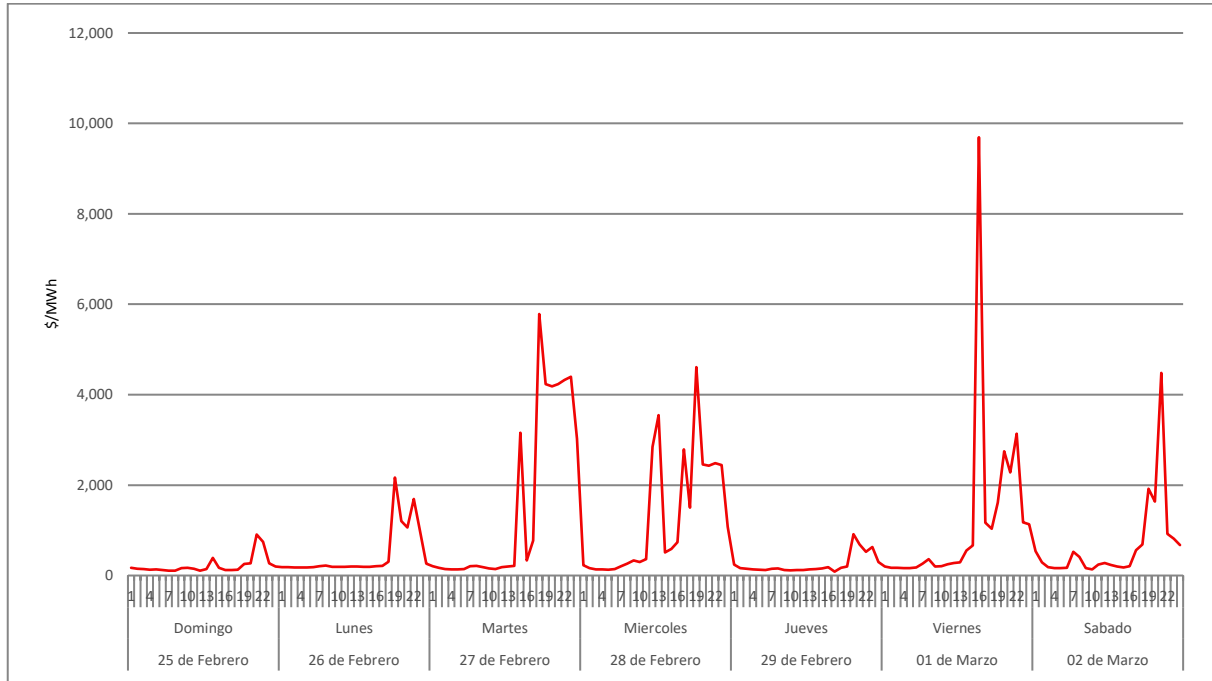
Figura 16. Precio de la Reserva de Regulación Secundaria de Frecuencia.
