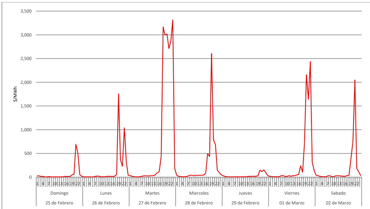
Figura 17. Precio de la Reserva Rodante de 10 minutos.
