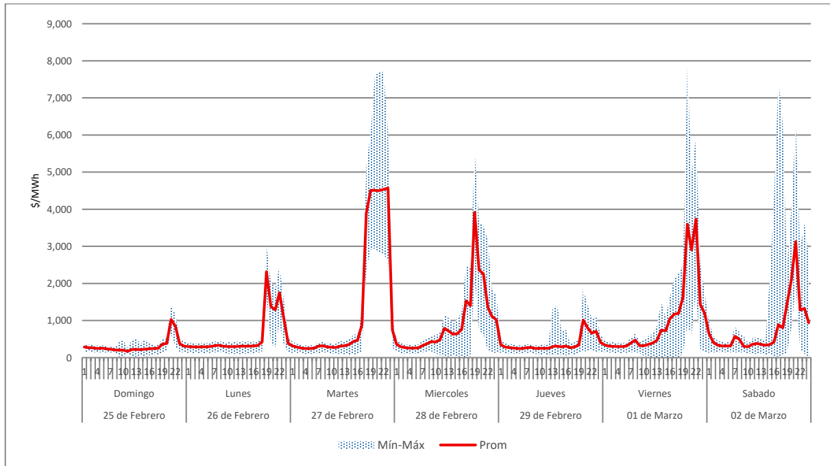
Figura 13. Precio Marginal Local Promedio en el MTR ex-post.
